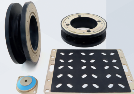
Titreşim Sönümleyici Grubu Vibration Dampening Products
